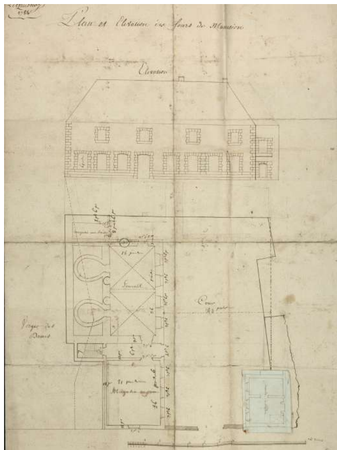
1784 - Plan et élévation du four de Monsion FRAD059_66J_183502A, Service Historique de la Défense
